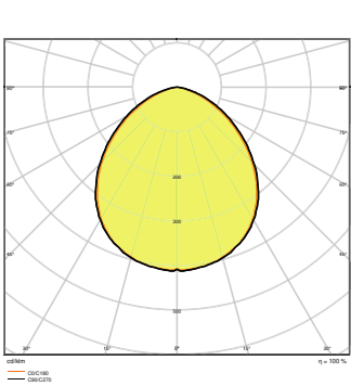
FL PFM 50W4000K SYM 100 S WT
