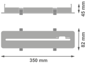
EM EXIT RECESSED KIT
