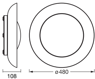
ORBIS PLATE 480 45W830CLICKDIM
