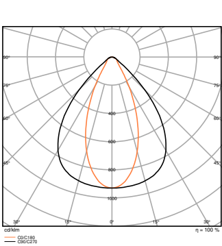
LB FLEX 1500 P 73W 840 OV
