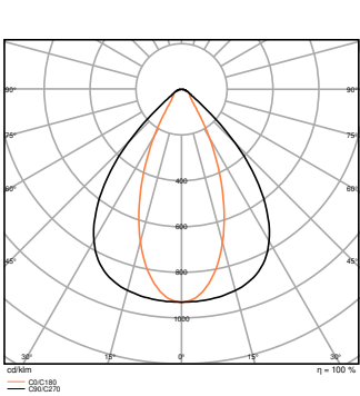
LB FLEX 1200 P 73W 840 OV
