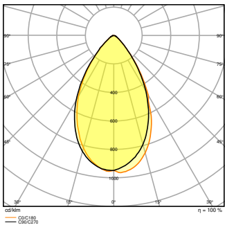
FL MAX LUM P 600W 757 SYM 60 WAL
