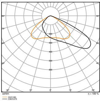
FL FLEX DA P 80W 840 A55X120 WAL LEDV
