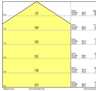
PL CMFT 600 P 28W 830 DALIVR EM
