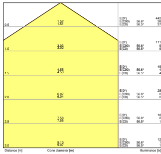
PL CMFT 600 P 28W 830 DALIVR EM CONVERSION BOX
