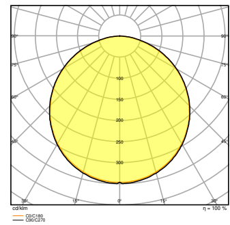
PL CMFT 600 P 28W 830 DALIVR
