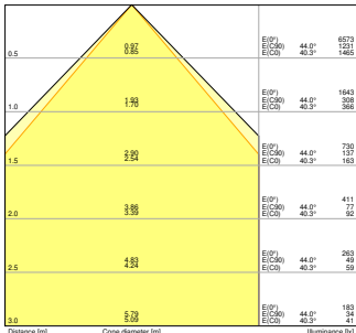
PL CMFT 600 P 25W 840 U19 PS
