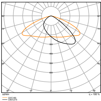
FL PFM DA 150W 4000K ASYM 45X140 BK
