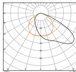
FL PFM 150W 4000K ASYM 55X110 BK
