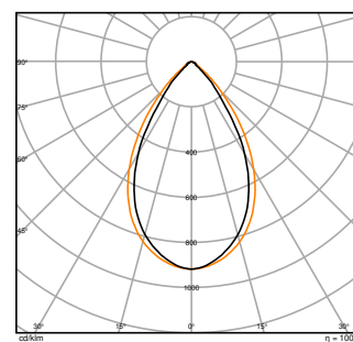
LB FLEX 1500 P 73W 840 N
