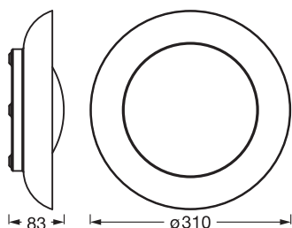
ORBIS PLATE 310 19W830CLICKDIM
