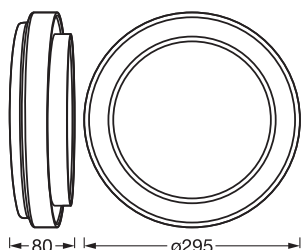
ORBIS RAZON 295MM 16W 830
