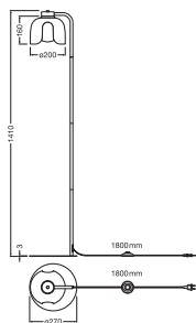
DECOR COROLLE FLOOR E27
