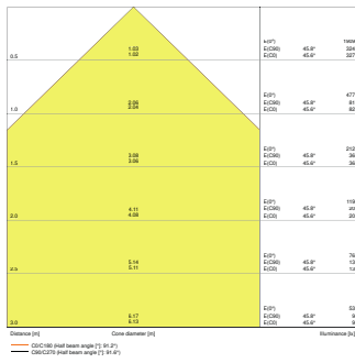
FL PFM 10W3000K SYM 100 BK
