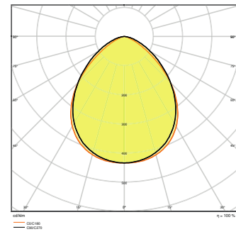
FL PFM 10W3000K SYM 100 BK
