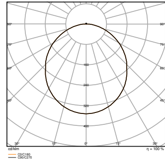
BLKH 250 P 8.5W 840 1070lm
