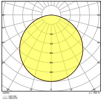
PL CMFT 625 P 33W 840 DALIVR
