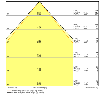
PL CMFT 600 P 28W 840 U19 DALIVR EM CONVERSION BOX
