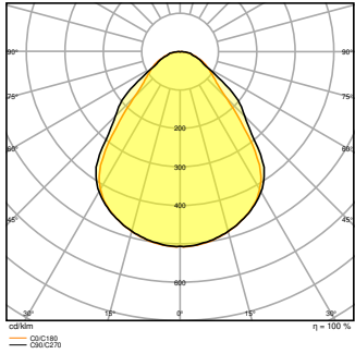
PL CMFT 600 P 28W 840 U19 DALIVR
