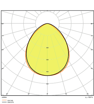
FL PFM 10W3000K SYM 100 S WT
