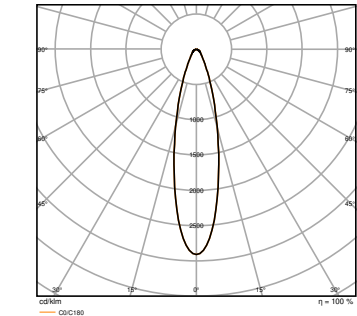
FL PFM 150W 3000K SYM R30 BK
