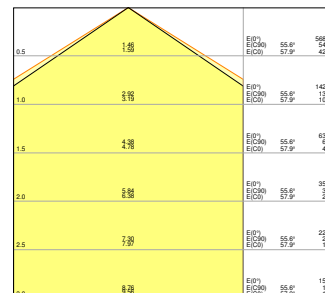
PL CMFT 1200 P 33W 840 DALIVR
